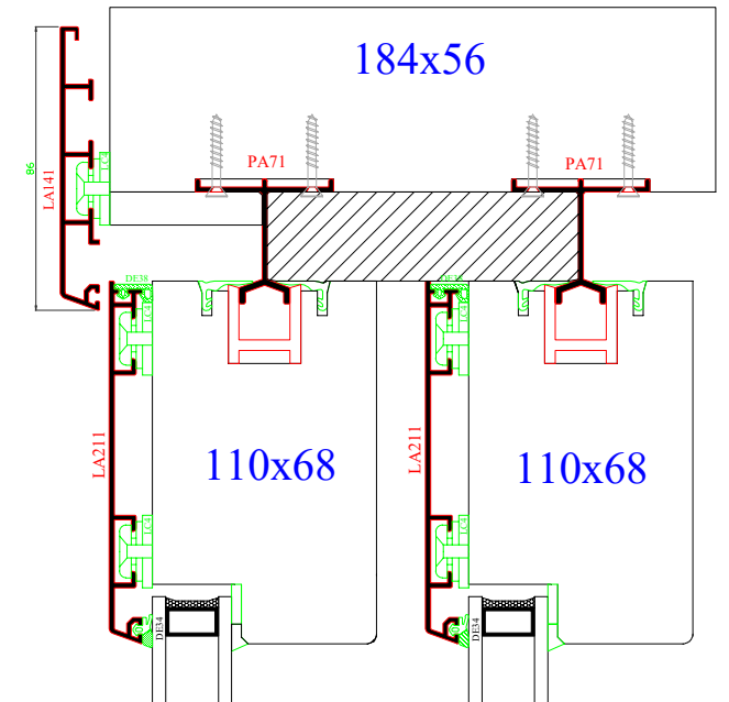
Coupe F
