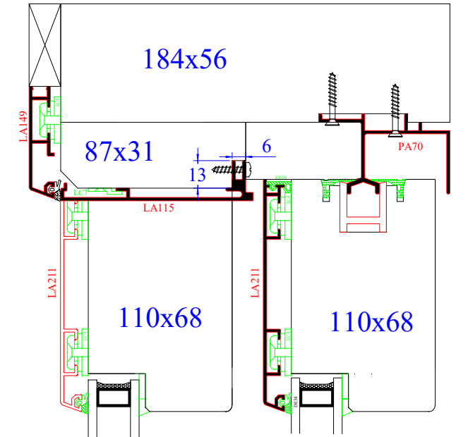
Coupe F
