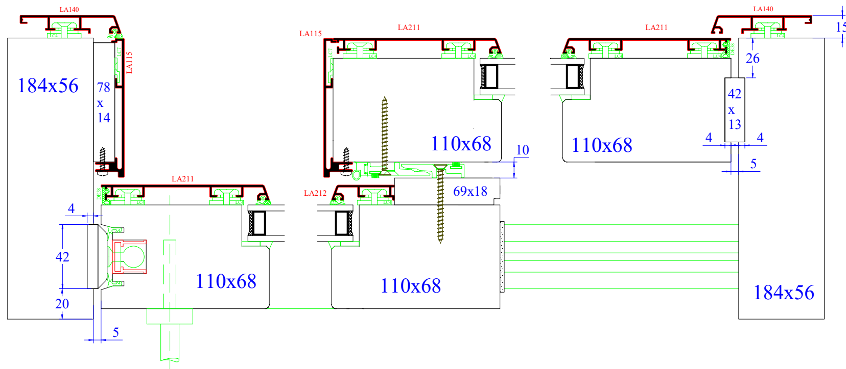
Coupe B
