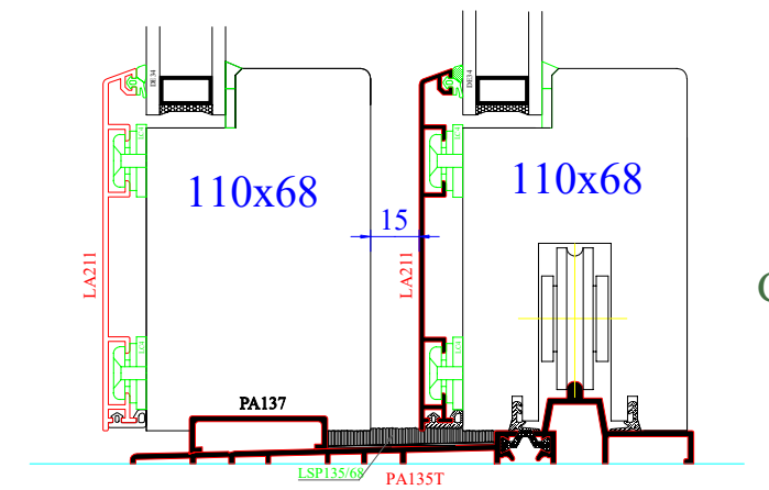
Coupe G
